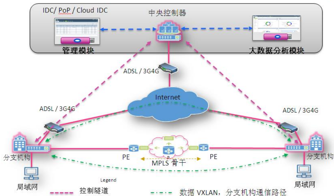
图 1: SD-WAN 物理架构
